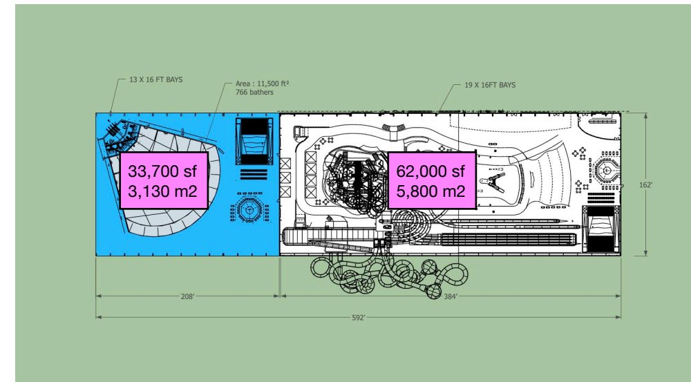
Expansion Option 2 ADD: Outdoor Wave Pool MED + Surf
